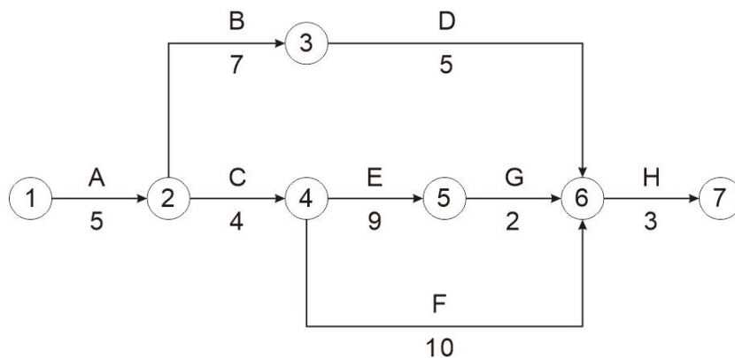
图3-1施工进度计划网络
