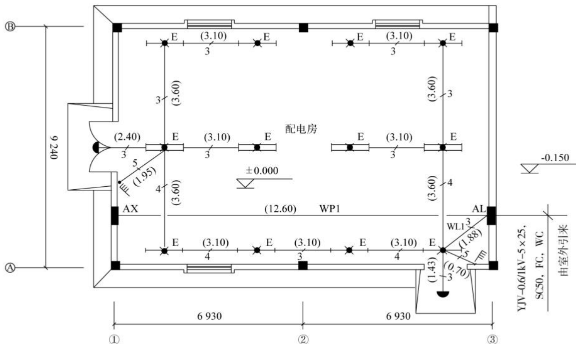
图 6. III. 1 配电房电气平面图
