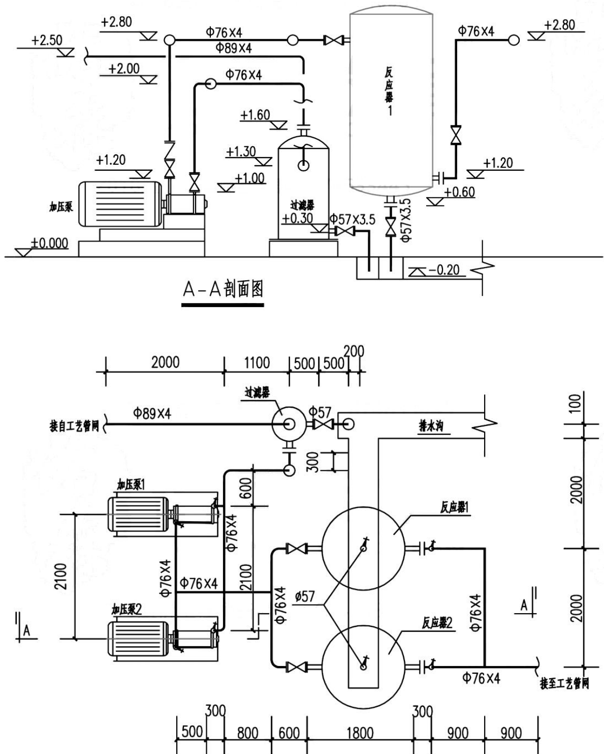
图3-5工艺管道系统
